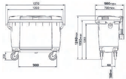
• Medidas de tachos LXD1100
