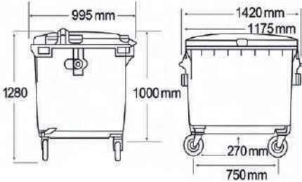
• Medidas de tachos LXD1100
